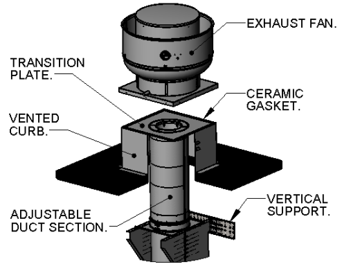
Fig. 8 – Fan Adapter Plate
